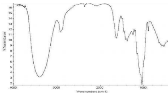
Gambar 4. Grafik Serapan FTIR Hemicelulosa Tongkol Jagung [17]
