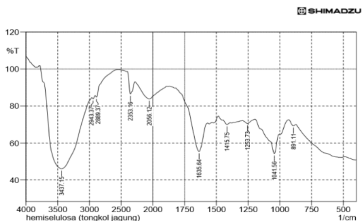
Grafik 3. Serapan FTIR Hemicelulosa Tongkol Jagung (Hasil isolasi)
